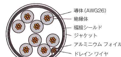
STP構造図(2重シールド)
