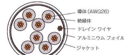
FTP構造図(1重シールド)
